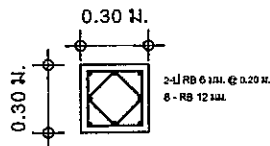
ขยายเสา
