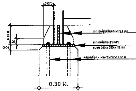
ขยายการต่อเชื่อมกับเสา ค.ส.ก.
