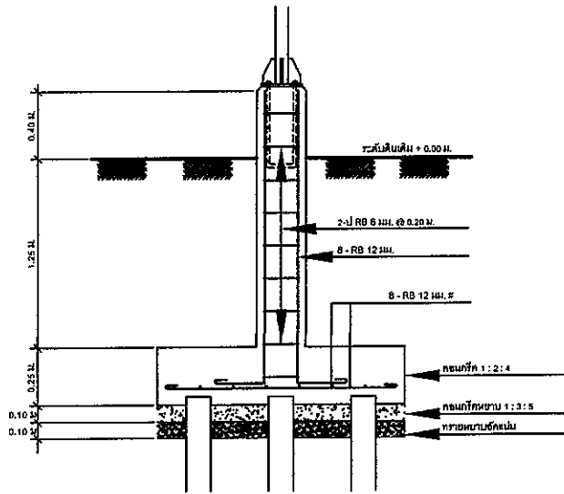
แปลนขยายฐานราก ขนาดจริง
