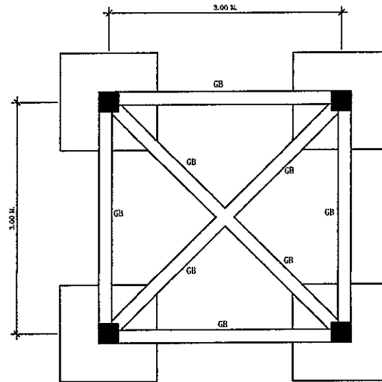
แปลนฐานราก ตามชนิด
