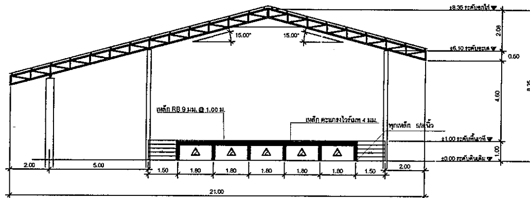
รูปตัด B
