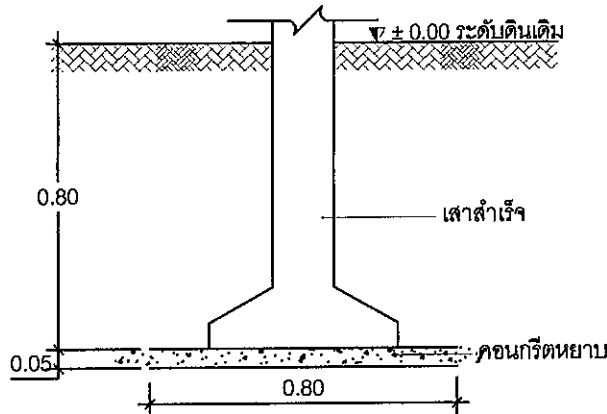
รูปตัดฐานราก F1
