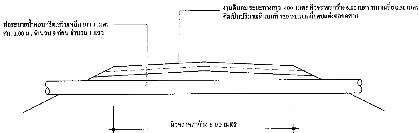
รูปตัดก่อสร้างถนนดินภายในหมู่บ้าน บ้าน โนนงาม หมู่ที่ 4
