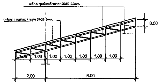
แปลนขยาย TRUSS 1 NTS
