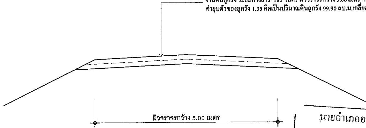
รูปตัดก่อสร้างถนนลูกรังภายในหมู่บ้าน บ้านนาเรือง หมู่ที่ 7 ช่วงที่ 2
