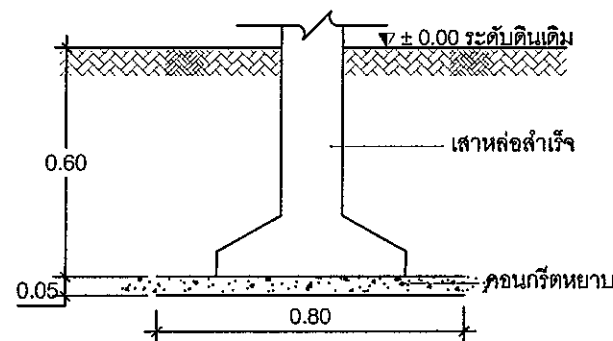
รูปตัดฐานราก F1
