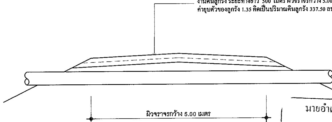
รูปตัดก่อสร้างถนนลูกรังภายในหมู่บ้าน บ้านม่วงโป้ หมู่ที่ 1
