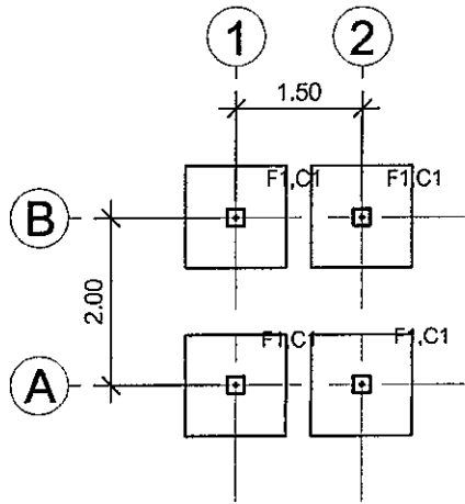
แปลนฐานราก มาตราส่วน 1 : 100
