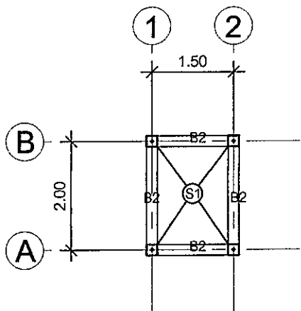
แปลนคาน มาตราส่วน 1 : 100
