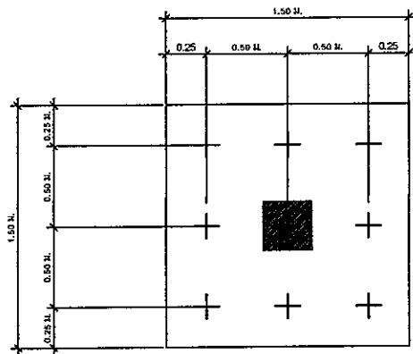
แปลนขยายฐานมาก
