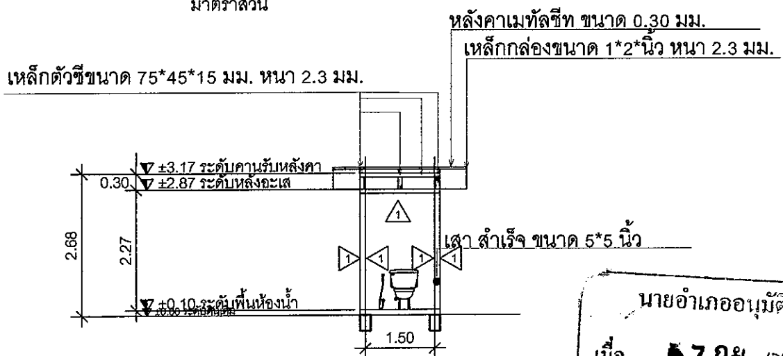
รูปตัด A มาตราส่วน
