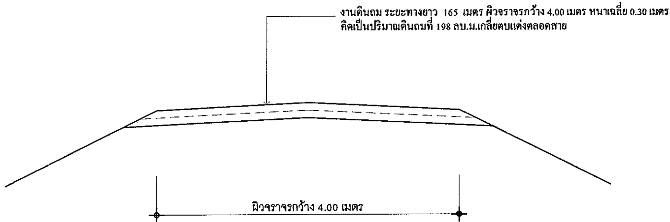
รูปตัดก่อสร้างถนนลูกรังภายในหมู่บ้าน บ้านนาเรือง หมู่ที่ 7 ช่วงที่ 1
