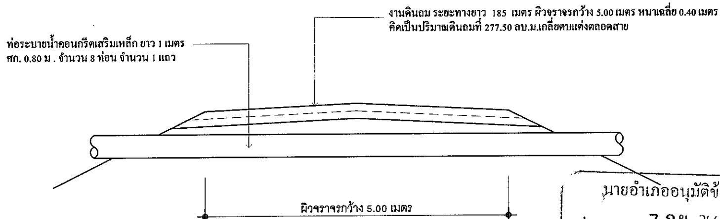
รูปตัดก่อสร้างถนนลูกรังภายในหมู่บ้าน บ้านนาเรือง หมู่ที่ 7 ช่วงที่ 2
