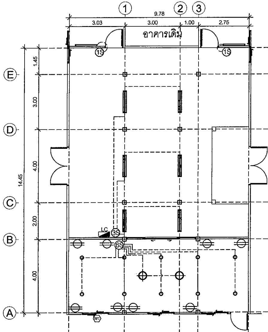
แปลนไฟฟ้า มาตราส่วน 1:125
