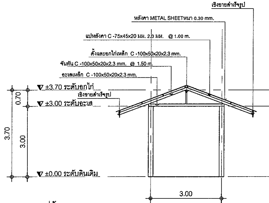
รูปตัด มาตราส่วน 1 : 100
