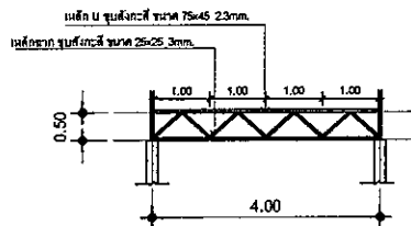
แปลนขยาย TRUSS 2 NTS
