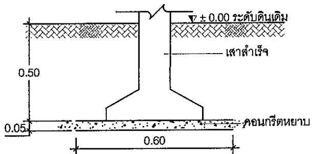
รูปตัดฐานราก F1 มาตราส่วน nts
