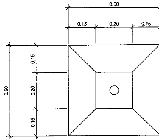
แปลนขยายฐานราก
