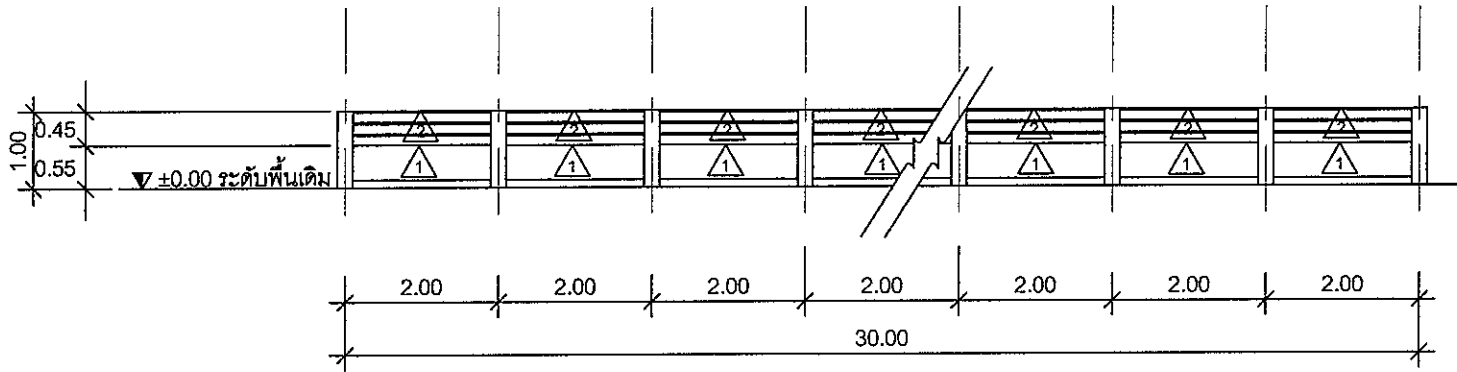
รูปด้าน มาตราส่วน 1 : 100
