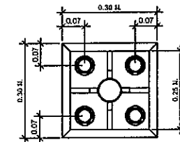
ขยายการต่อเชื่อมกับเสา ค.ส.ก.
