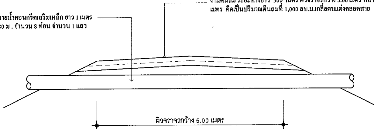
รูปตัดก่อสร้างถนนลูกรังภายในหมู่บ้าน บ้านม่วงโป้ หมู่ที่ 1
