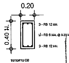
ขยายฐาน GB
